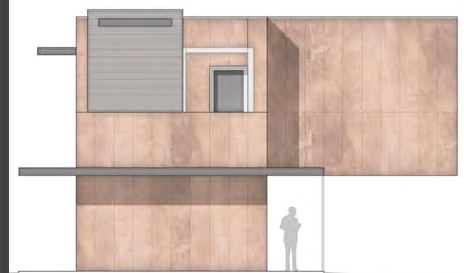
PROSPETTO OVEST
