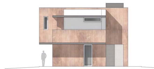
PROSPETTO SUD
